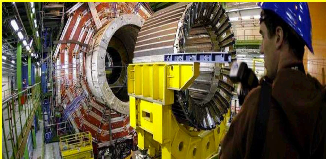
IL C.E.R.N.: COL PIÙ GRANDE ACCELERATORE DI PARTICELLE DEL MONDO, L'“L.H.C.”
