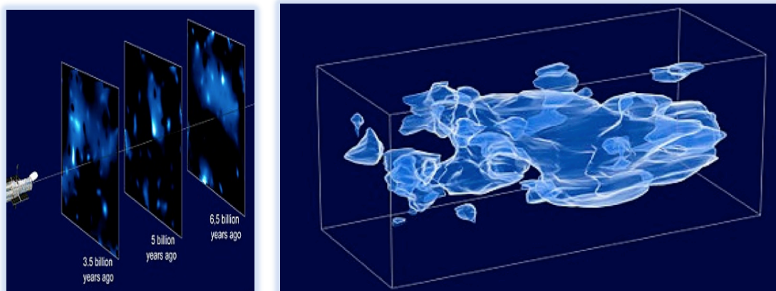
MAPPA DI “MATERIA OSCURA” TRACCIATA DAL TELESCOPIO SATELLITARE “HUBBLE”
