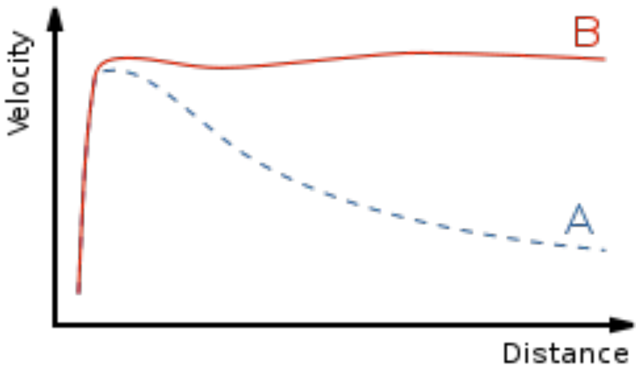
CURVA DI ROTAZIONE DELLA “GALASSIA SPIRALE”: (A)= CALCOLATA/PREVISTA; (B)=OSSERVATA.
